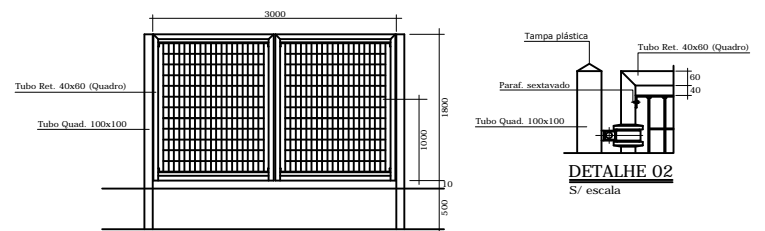
DETALHE DOS PORTÕES S/ escala
