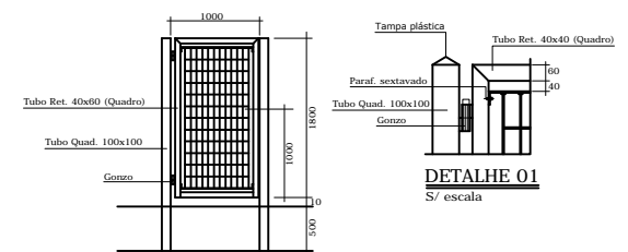
DETALHE DOS PORTÕES S/ escala
