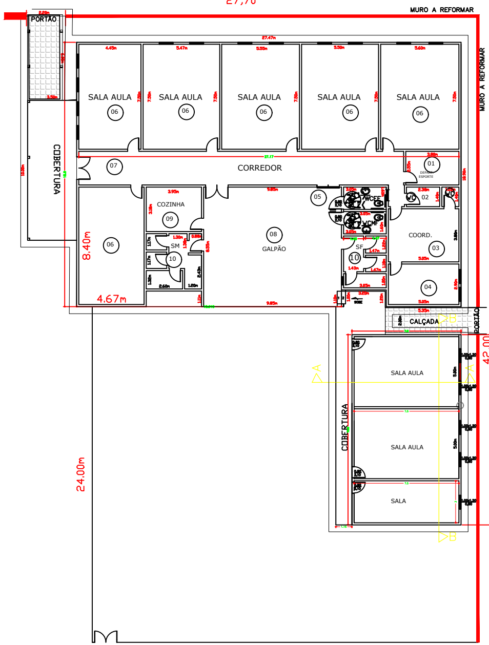
PLANTA BAIXA - Esc. 1:100
