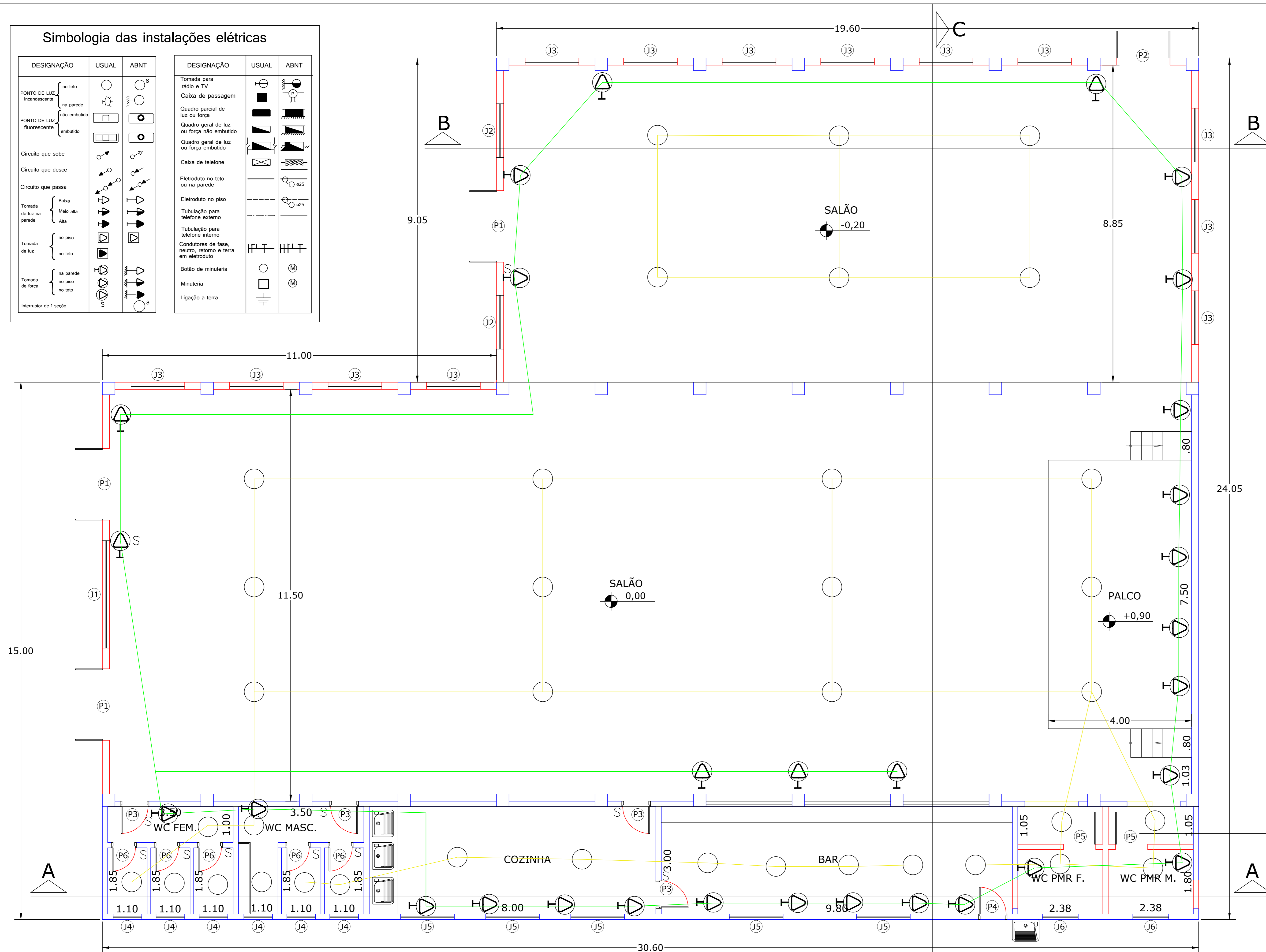
PLANTA BAIXA ESC. 1:100
