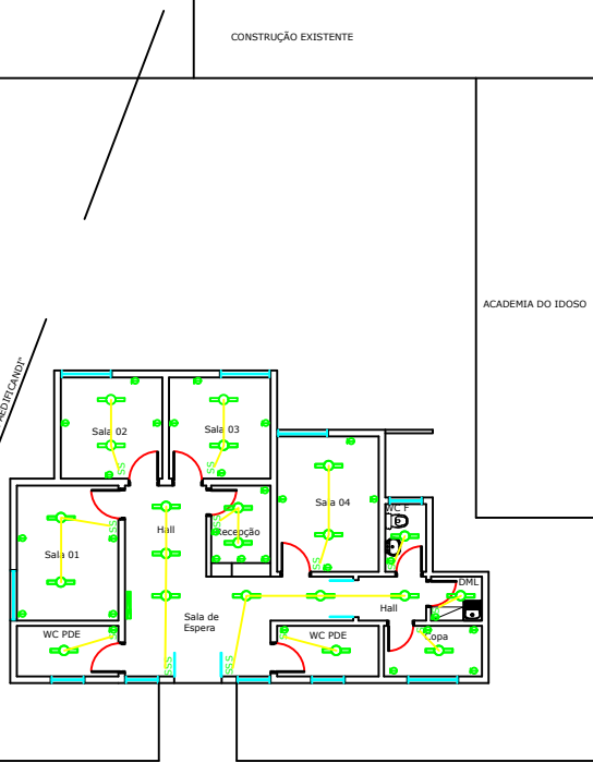
PLANTA BAIXA (AMPL. SALAS MULTIUSO) Escala 1:100
