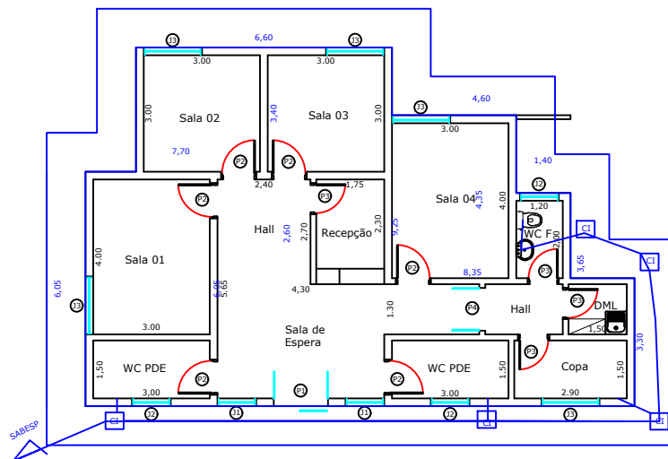
PLANTA BAIXA (AMPL. SALAS MULTIUSO) Escala 1:100
