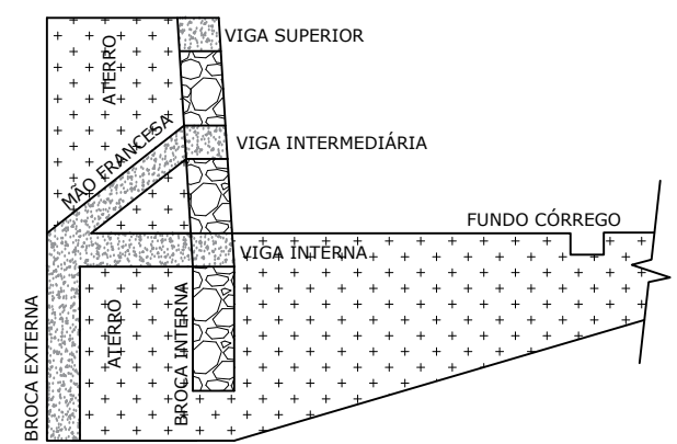
CORTE MURO CATANDUVA
