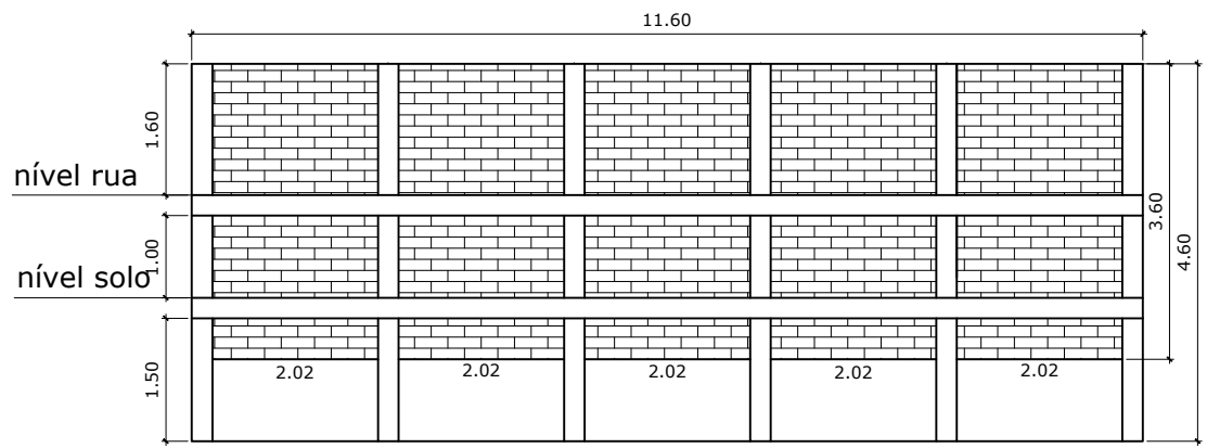
MURO DE ALVENARIA KAN
