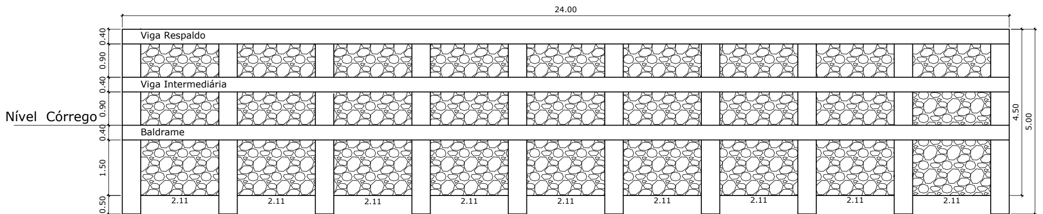
Muro de Arrimo Catanduva 10 Brocas 1,5 x 0,50 x 0,40
