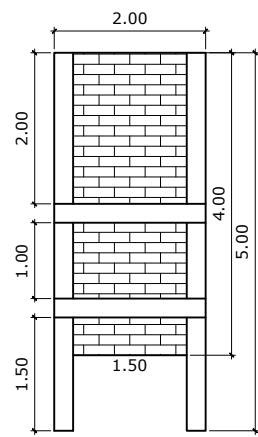
MURO DE ALVENARIA LOPES
