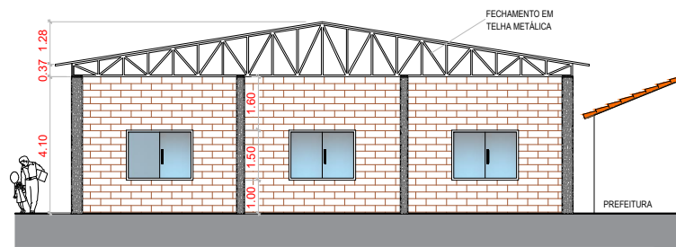
CORTE AA
