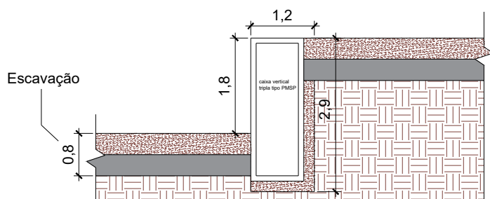
CORTE AA
