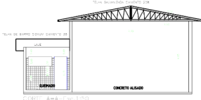
CORTE - AVA - Esc. 1:200
