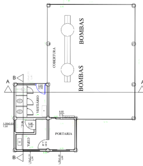
PLANTA BAIXA Esc. 1:50
