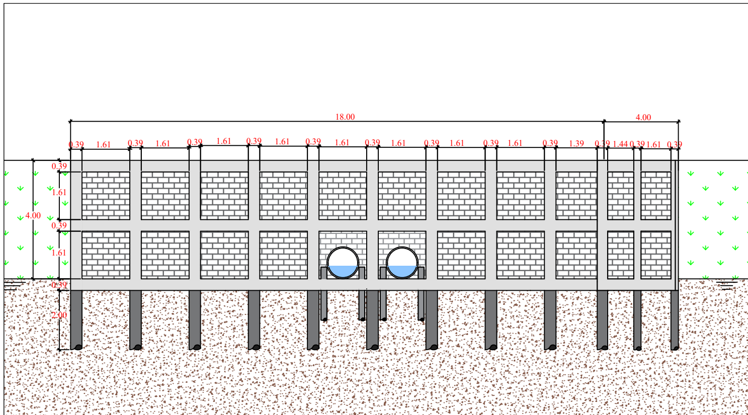
ELEVAÇÃO FRONTAL
