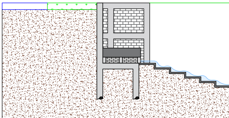
ELEVAÇÃO LATERAL
