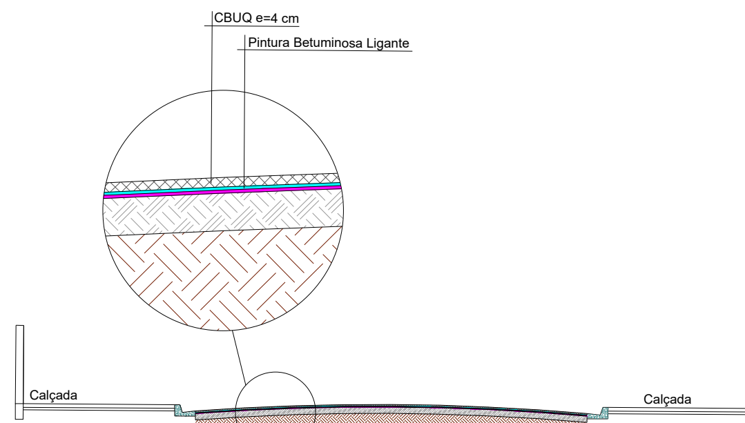
PERFIL TRANSVERSAL RECAPEAMENTO ESCALA 1:100
