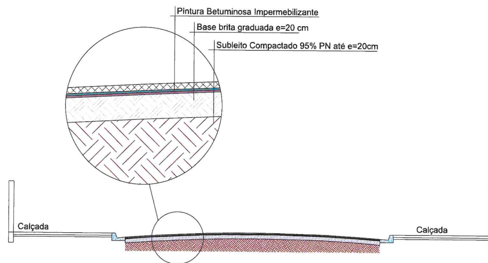
PERFIL TRANSVERSAL RECUPERAÇÃO DE BASE ESCALA 1:75
