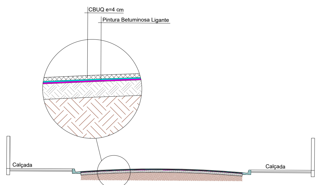
PERFIL TRANSVERSAL RECAPEAMENTO ESCALA 1:100
