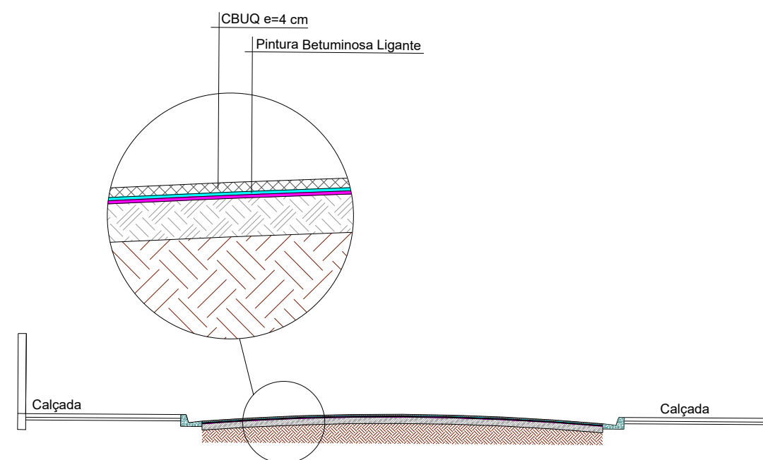
PERFIL TRANSVERSAL RECAPEAMENTO ESCALA 1:100
