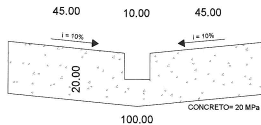
PERFIL DO SARJETÃO ESCALA 1:20
