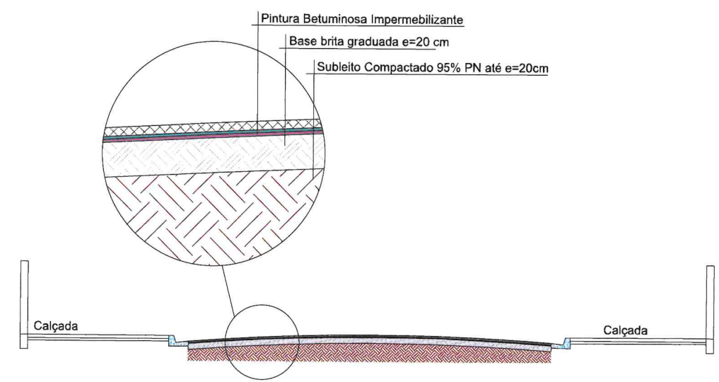
PERFIL TRANSVERSAL RECUPERAÇÃO DE BASE ESCALA 1:75
