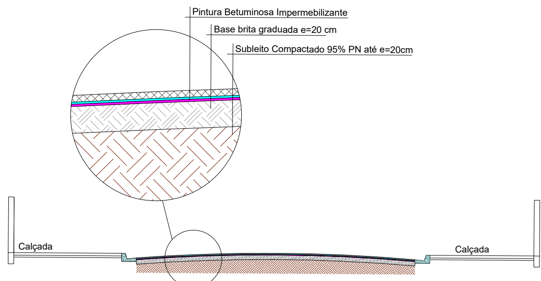
PERFIL TRANSVERSAL RECUPERAÇÃO DE BASE ESCALA 1:100
