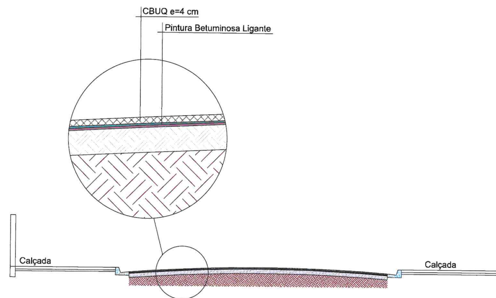
PERFIL TRANSVERSAL RECAPEAMENTO ESCALA 1:75
