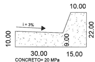
PERFIL DE GUIA E SARJETA ESCALA 1:20
