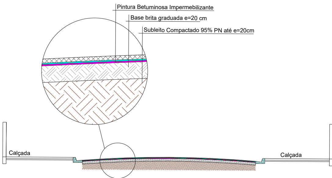
PERFIL TRANSVERSAL RECUPERAÇÃO DE BASE ESCALA 1:100
