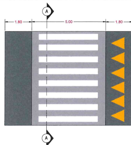
DETALHE LOMBOFAIXA ESCALA 1:100
