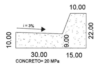
PERFIL DE GUIA E SARJETA ESCALA 1:20
