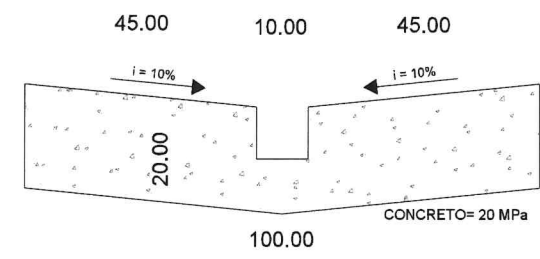
PERFIL DO SARJETÃO ESCALA 1:20
