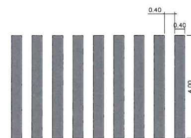
DETALHE FAIXA DE PEDESTRE ESCALA 1:100
